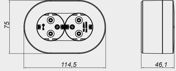
İKİLİ PRİZ
