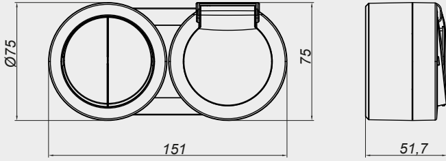
KOMÜTATÖR + KAPAKLI TOPRAKLI PRİZ
