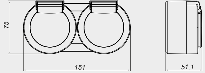
KAPAKLI TOPRAKLI PRİZ + KAPAKLI TOPRAKLI PRİZ
