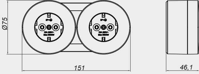
İKİLİ TOPRAKLI PRİZ
